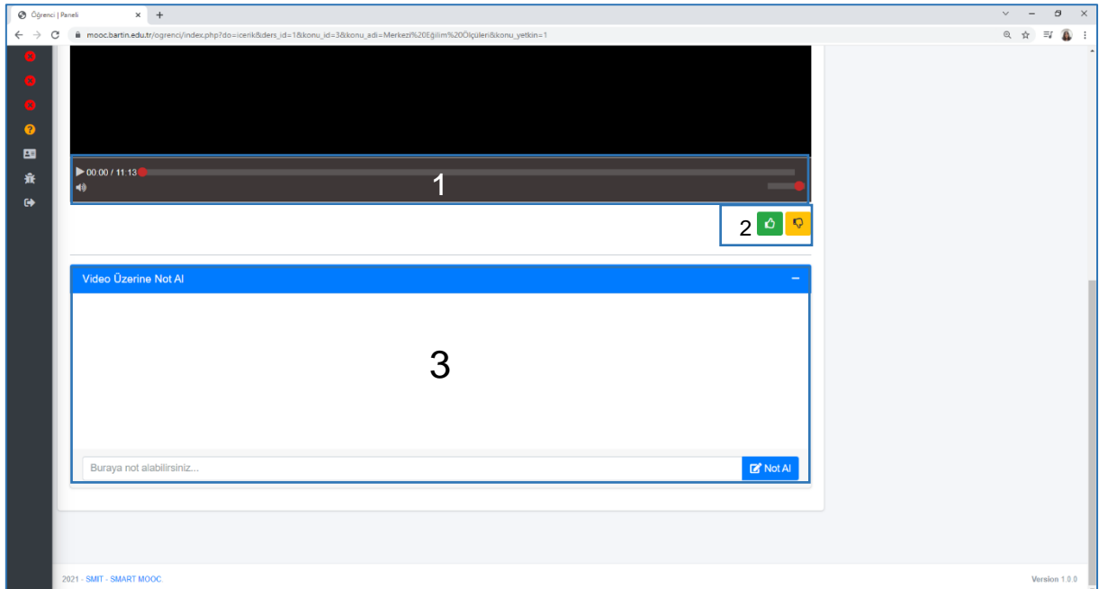
Şekil 14. Video etkileşimleri
